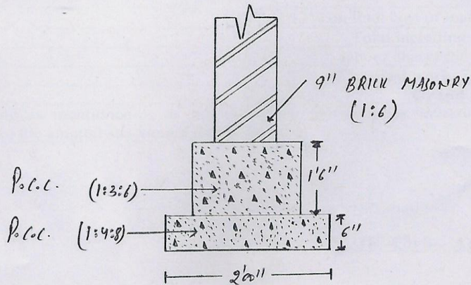
FIG. 2 ⇒ FOUNDATION DETAILS
